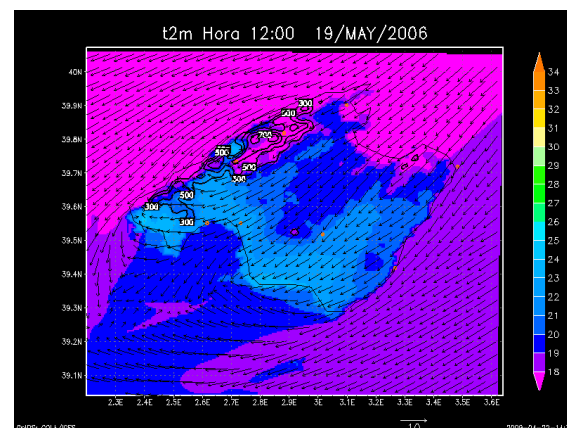
Figura 113. Ejemplo de no desarrollo de brisa
