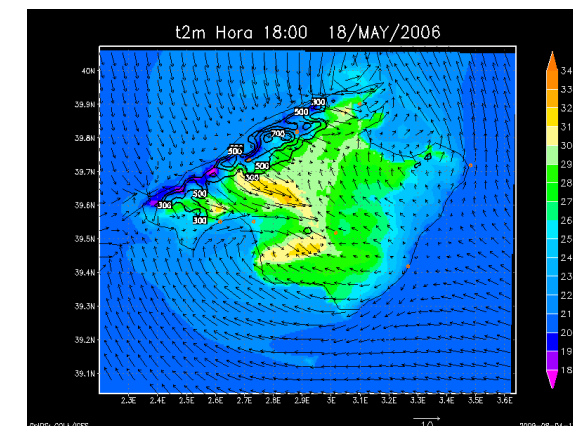
Figura 111. Ejemplo de día de brisa intensa a las 18 UTC
