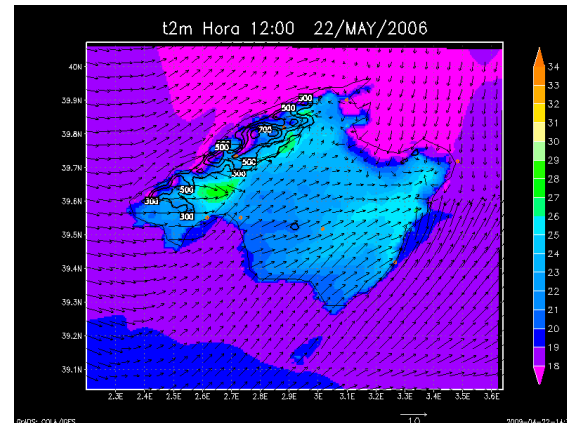
Figura 112: Ejemplo de brisa débil
