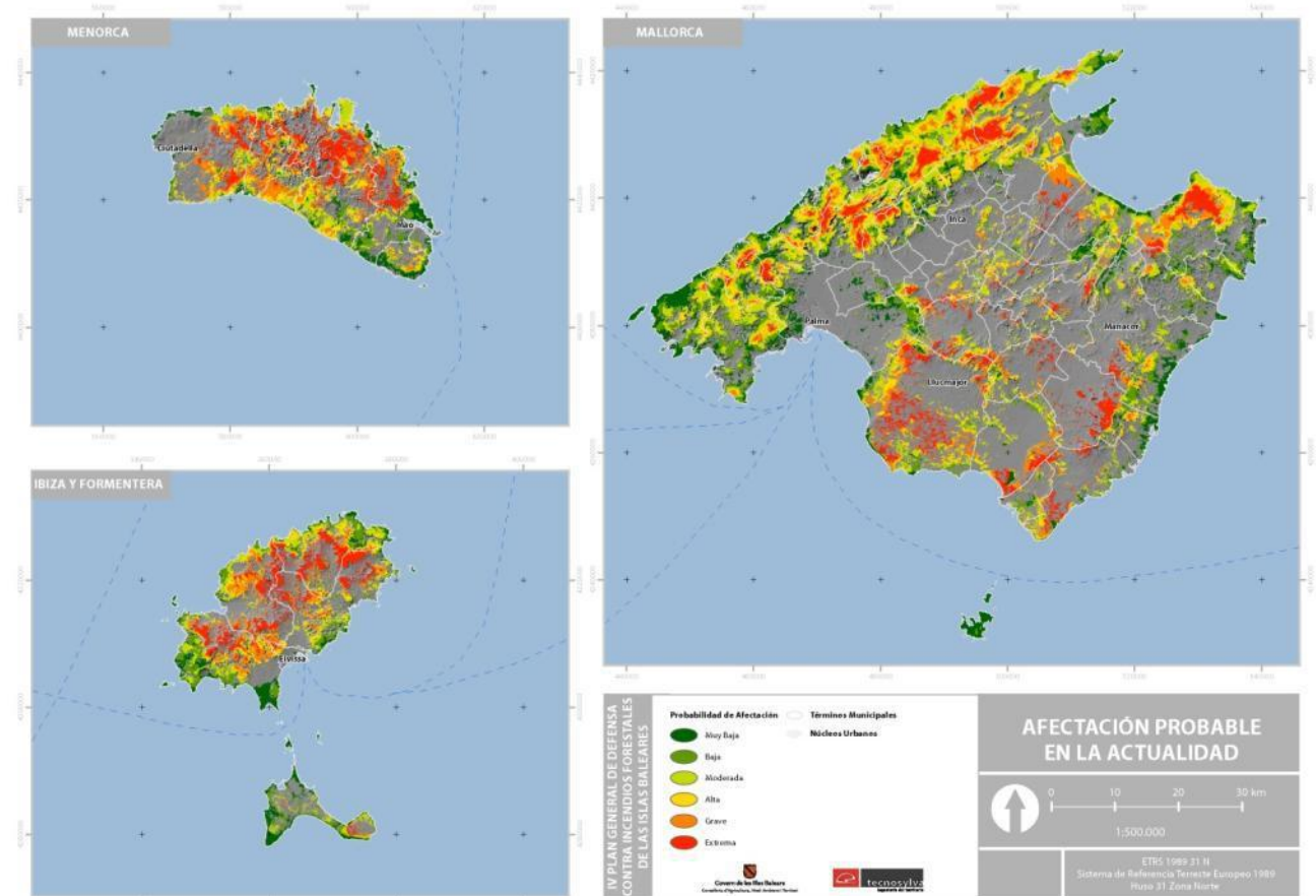
Figura 207: Resultado de la simulación probabilística para 4000 puntos de ignición en el escenario actual
