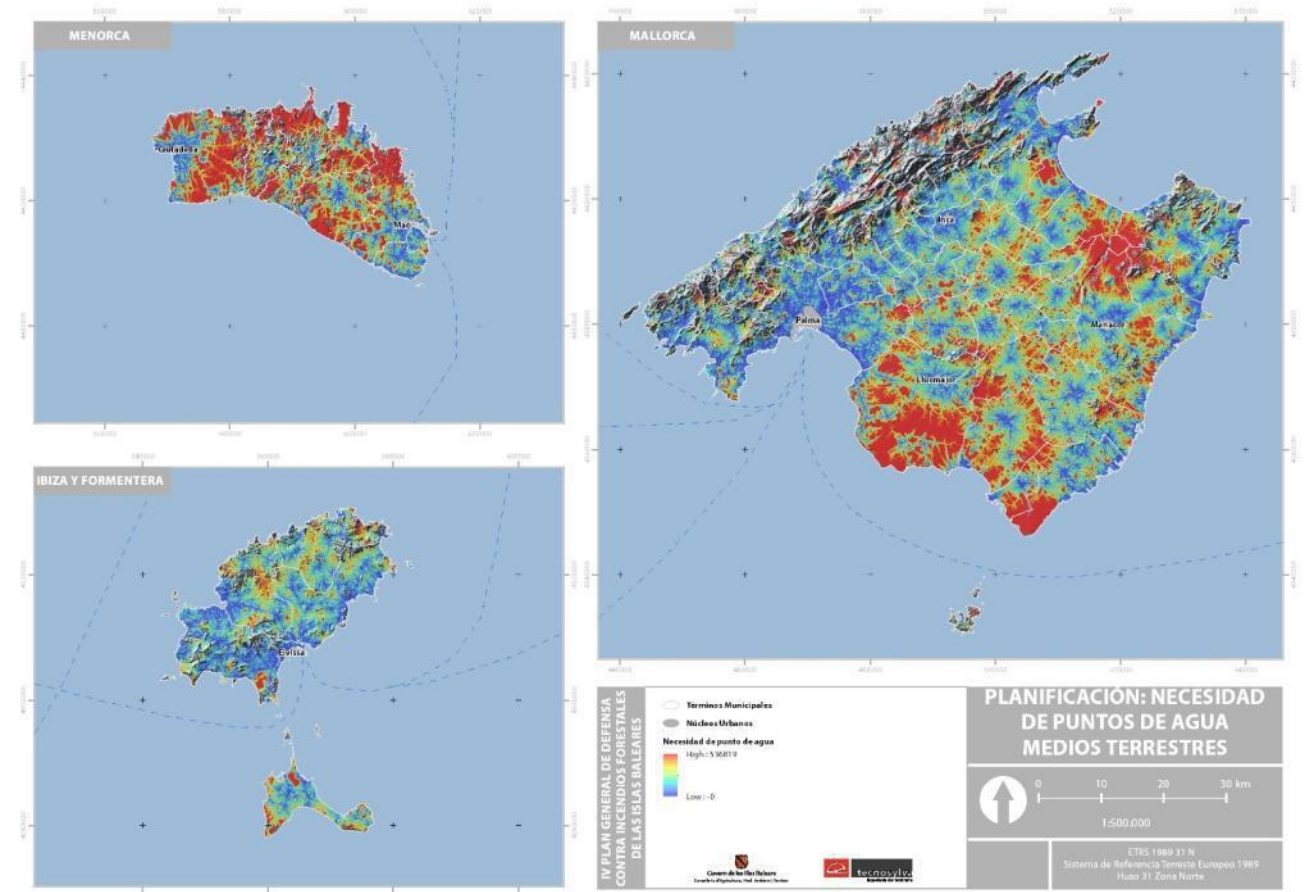
Figura 201: Necesidades de construcción de nuevo punto de agua para medios terrestres
