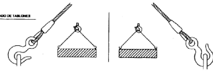
CARGA CON DOS ESLINGAS SIN FIN
