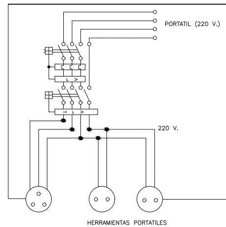
Cuadro con protección frente a cortocircuitos y corrientes de defecto. Se instalará en las plantas o zonas en donde se precise su utilización. ESQUEMA UNIFILAR DEL CUADRO AUXILIAR ELECTRICO DE OBRA PARA MAQUINARIA PORTATIL.
