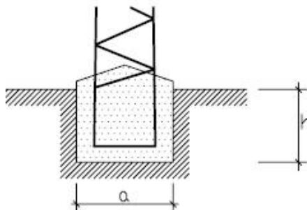
Cimentación monobloque
