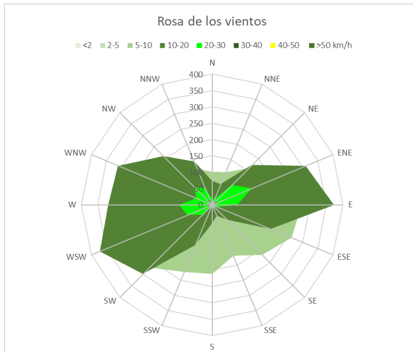
Ilustración 8.- Rosa de los vientos.
