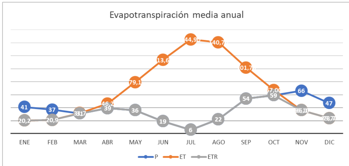
Ilustración 6.- Evapotranspiración.
