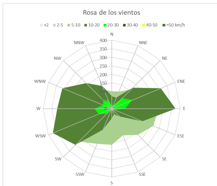
Ilustración 20.- Rosa de los vientos de Palma de Mallorca. Fuente: Elaboración propia.
