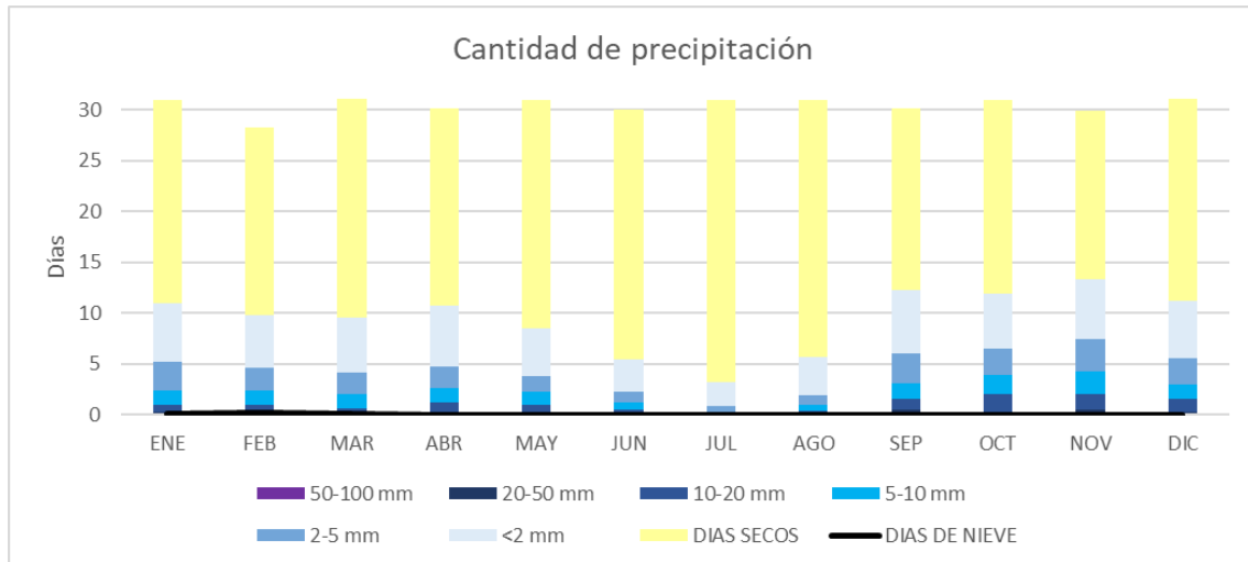
Ilustración 5.- Precipitación.
