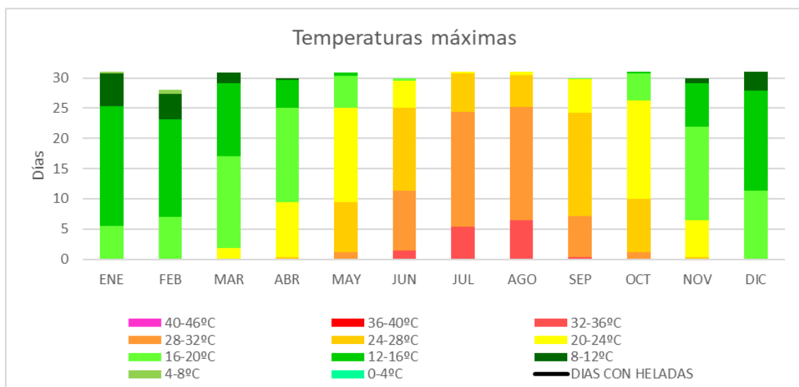
Ilustración 4.- Temperaturas máximas.
