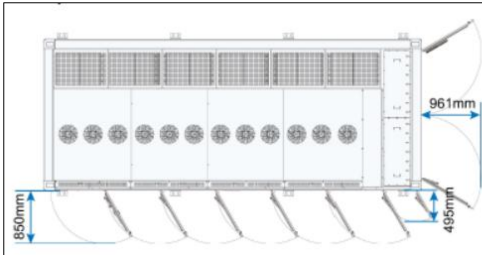
Imagen 40. Distancias mínimas para el mantenimiento.
