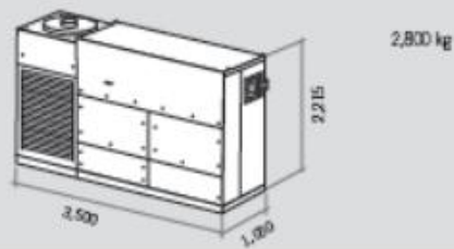
Imagen 15. Detalle de los inversores.
