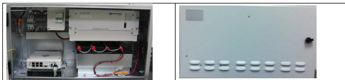
Imagen 33. Equipo rectificador-cargador de baterías
