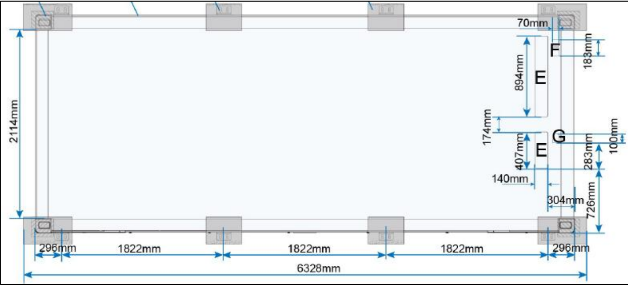
Imagen 36. Cimentaciones propuestas.
