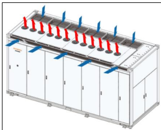
Imagen 39. Sistema de ventilación incorporado.
