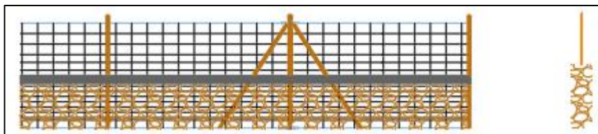
Imagen 35. Detalle del cerramiento de la parcela
