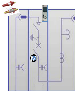
Imagen 21. Unidad de protección ekorRPA-220
