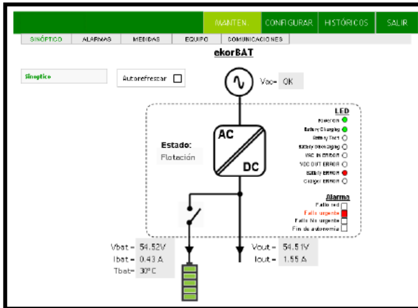
Imagen 34. Esquema ekorBAT
