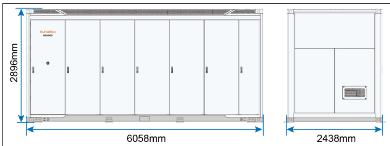
Imagen 11. Container de baterías.
