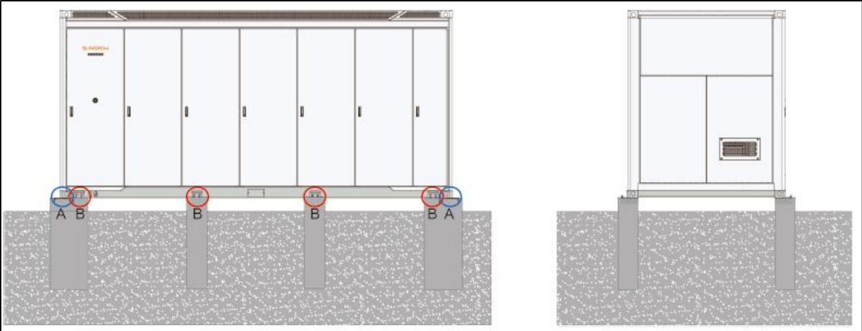
Imagen 37. Sección de las cimentaciones.
