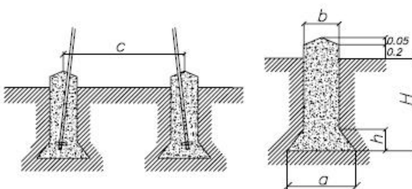
Cimentación tetrabloque cuadrada o circular con cueva
