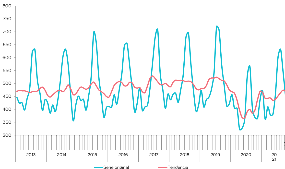
Gráfico 8. Energía eléctrica mensual demandada en las Islas Baleares (GWh)
