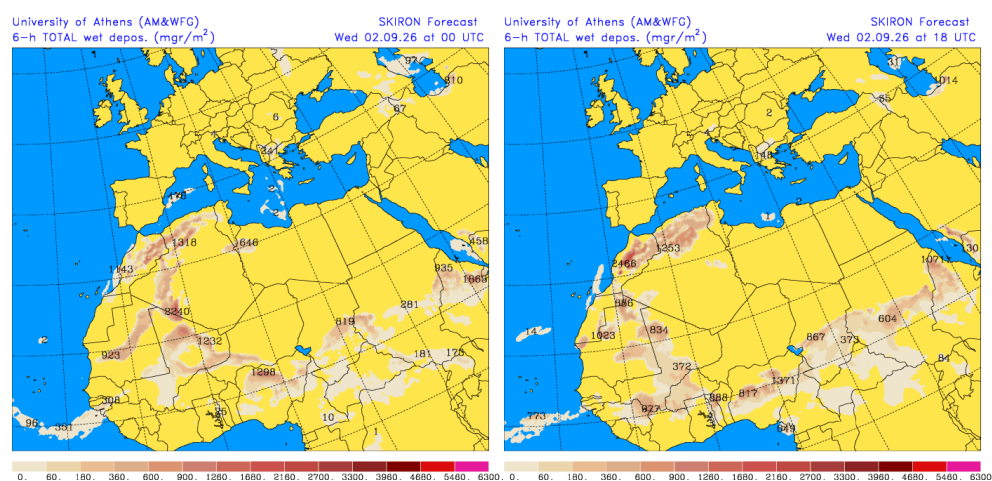
Depósito húmedo de polvo ( \text{mg}/\text{m}^2 ) predicho por el modelo SKIRON para el día 2 de septiembre de 2026 a las 00 y 18 UTC © Universidad de Atenas.
