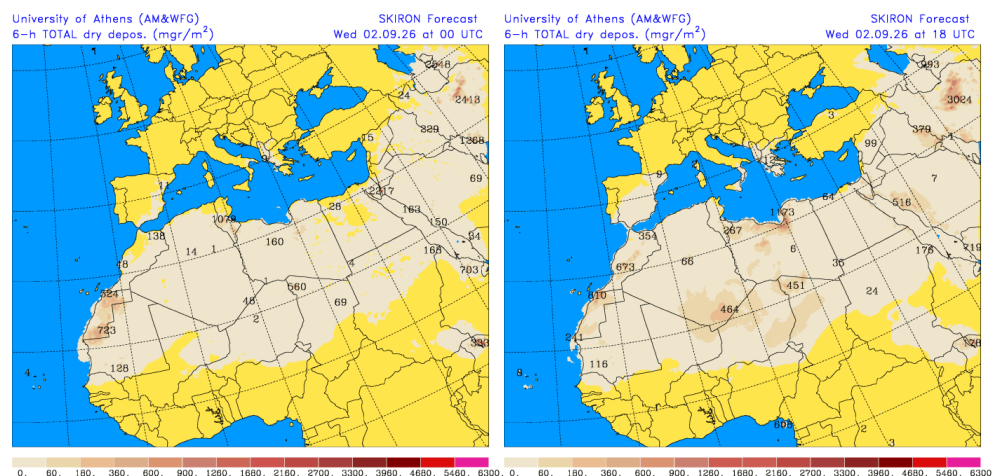
Depósito seco de polvo ( \text{mg}/\text{m}^2 ) predicho por el modelo SKIRON para el día 2 de septiembre de 2026 a las 00 y 18 UTC © Universidad de Atenas.
