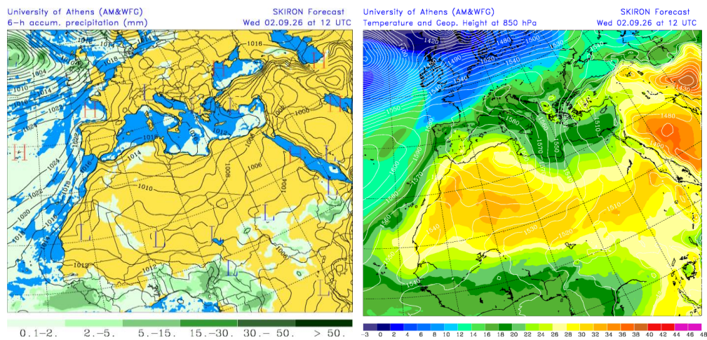
Precipitación acumulada (mm) y presión a nivel del mar (hPa) (izquierda) y campo de temperaturas (°C) y de altura geopotencial a 850 hPa (derecha) previsto por el modelo SKIRON para el día 2 de septiembre de 2026 a las 12 UTC © Universidad de Atenas.
