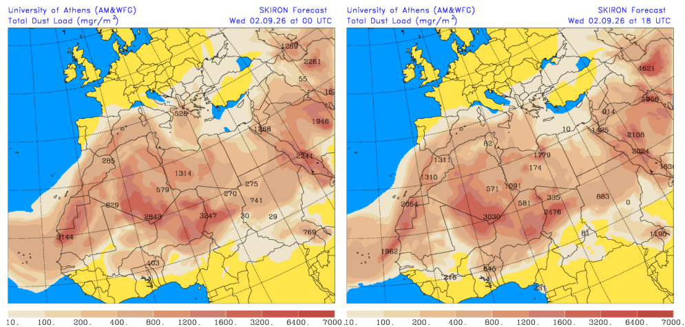
Carga total de polvo (mg/m 2 ) predicha por el modelo SKIRON para el día 2 de septiembre de 2026 a las 00 y 18 UTC © Universidad de Atenas.
